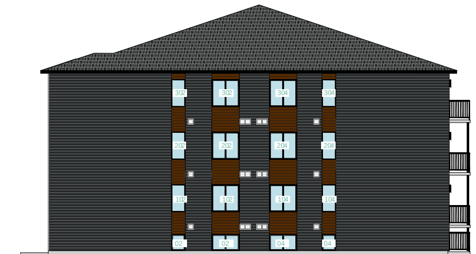
Élévation latérale droite
